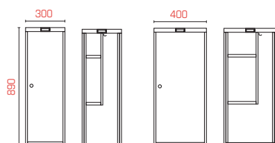
Helskåp SFXSL301* och SFXSL401*
