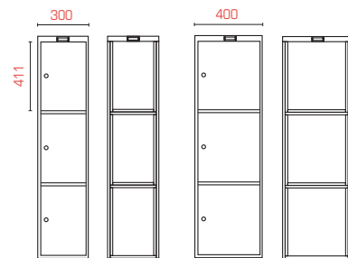
Tredjedelsskåp SFXSM303 och SFXSM403
