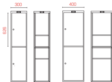
Halvskåp SFXSM302* och SFXSM402*
