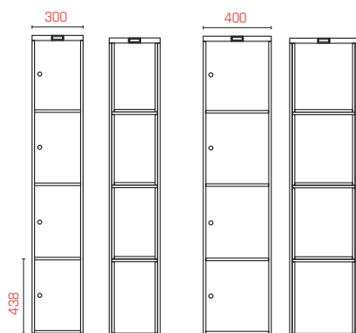
Fjärdedelsskåp SFXSH304 och SFXSH404
