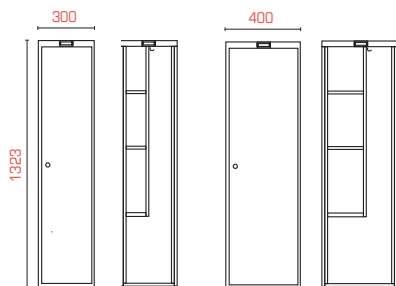
Helskåp SFXSM301** och SFXSM401**
