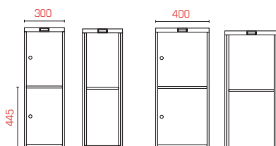
Halvskåp SFXSL302 och SFXSL402
