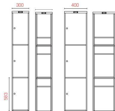
Tredjedelsskåp SFXSH303* och SFXSH403*
