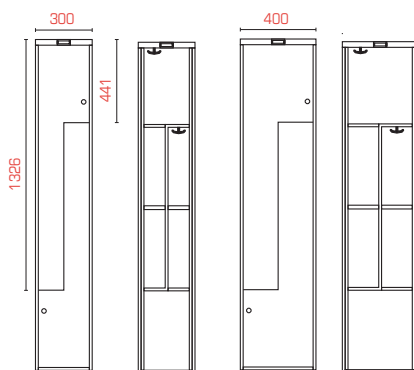
Z-skåp SFXSH3Z2 och SFXSH4Z2
