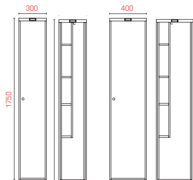
Helskåp SFXSH301** och SFXSH401**
