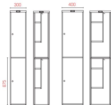
Halvskåp SFXSH302* och SFXSH402*
